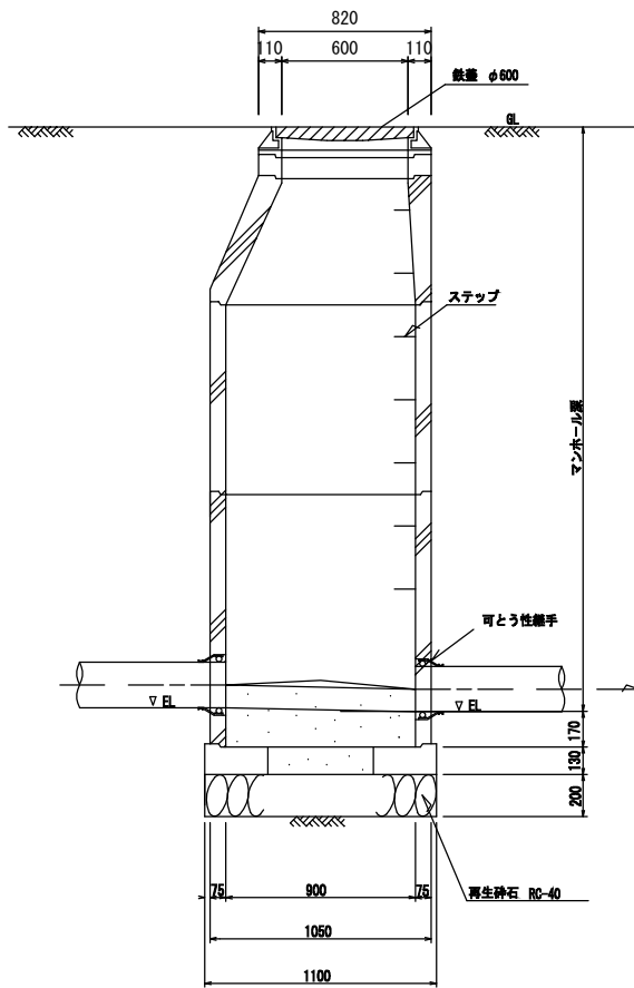
A-A断面図
