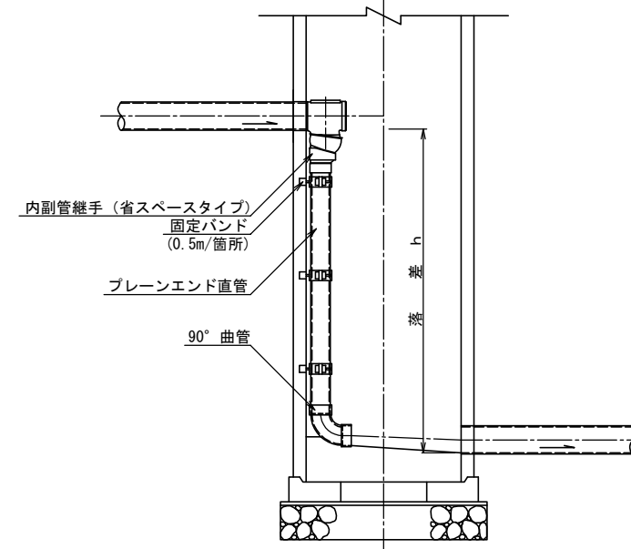
断面図
