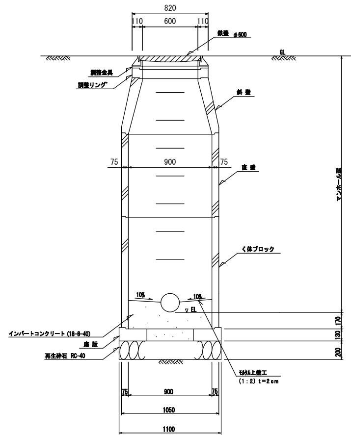
B-B断面図
